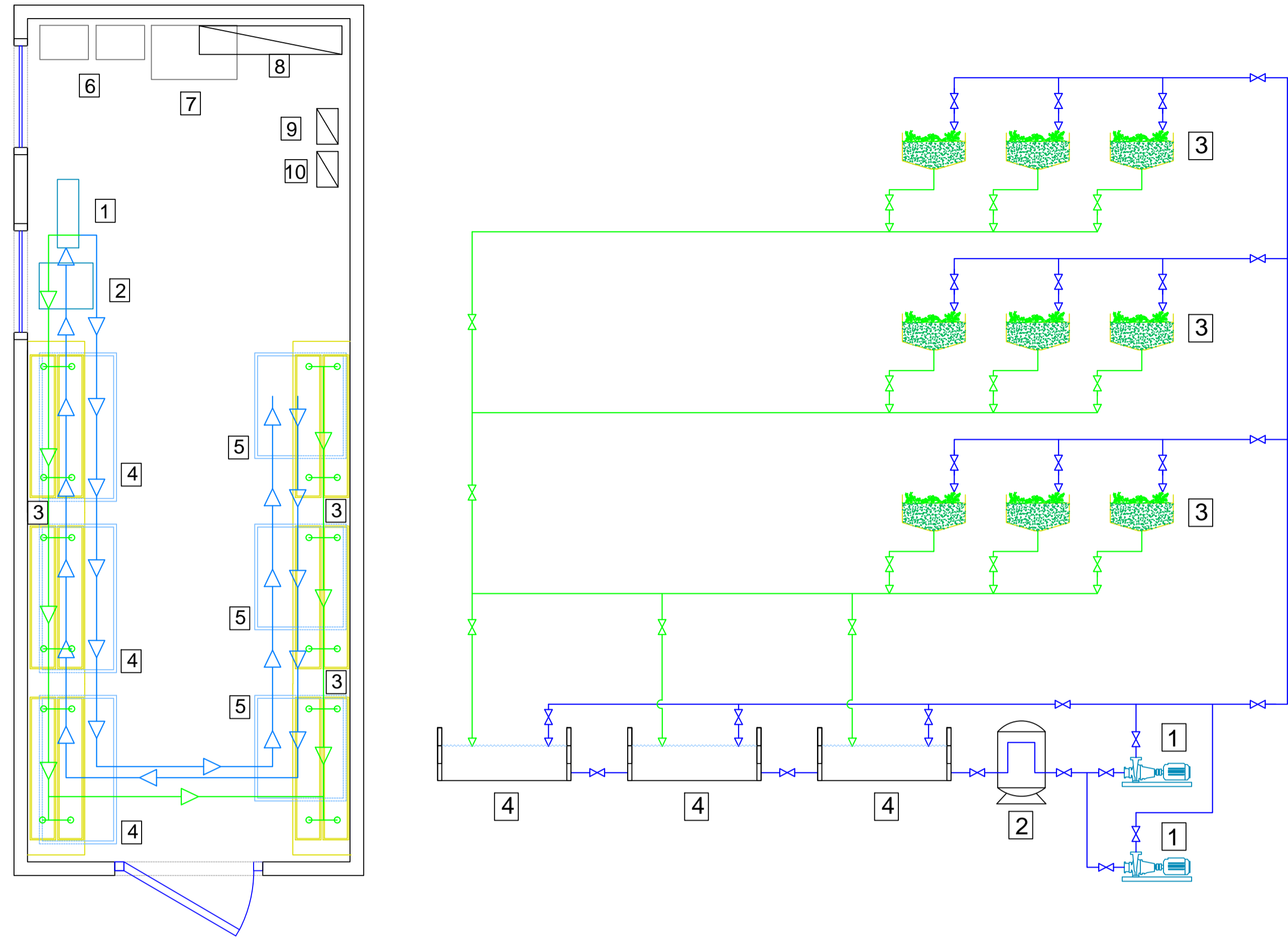
Planimetria Impianto idrico Cellula Vitale scala 1:25
